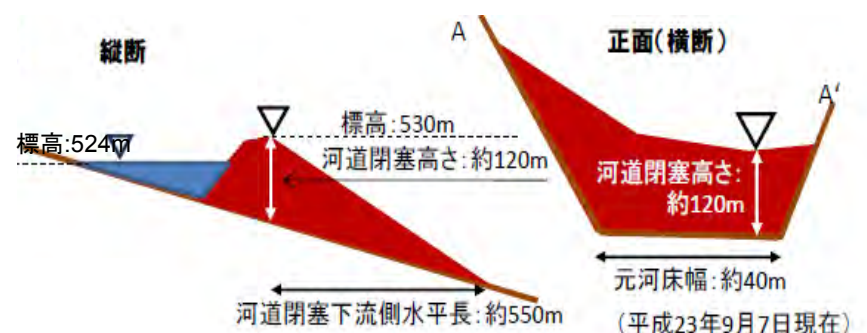
奈良県熊野川（十津川）流域 断面図 【↑上写真箇所】
