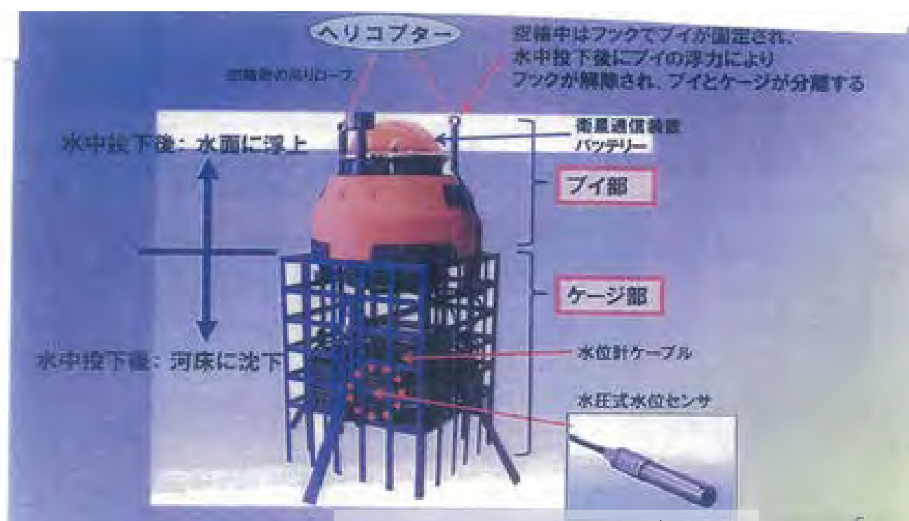
投下型水位観測ブイ
