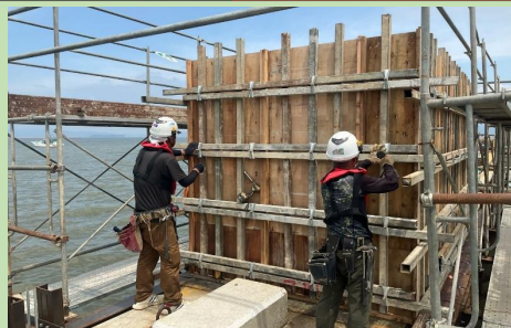
上部工型枠組立状況(4月下旬頃~8月頃) 予定
