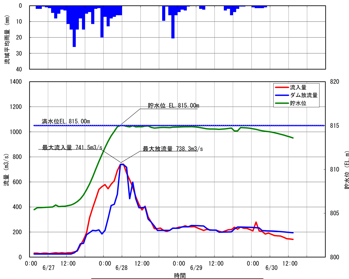
5 美和ダム洪水調節図 昭和36年6月28日洪水
