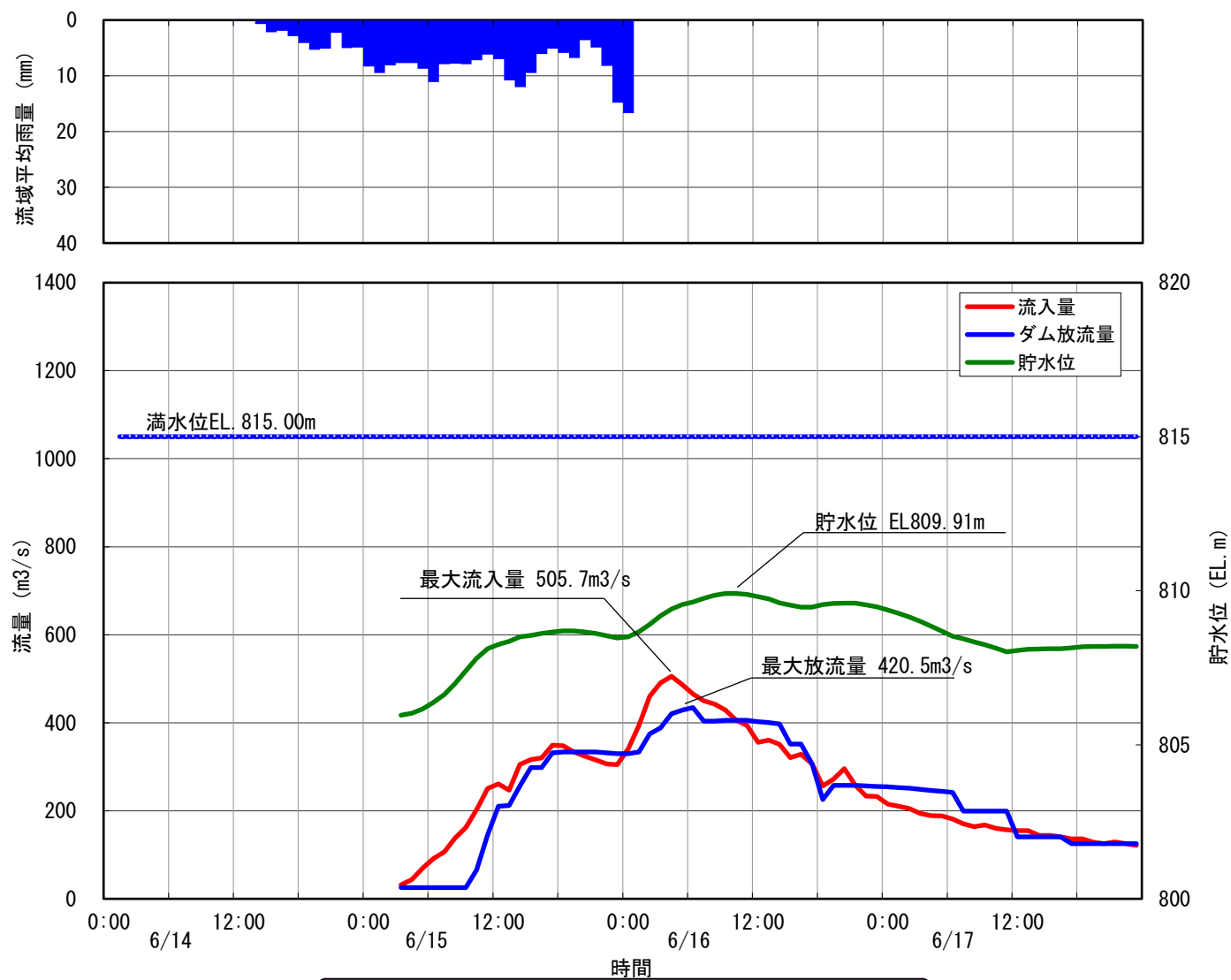
8 美和ダム洪水調節図 昭和45年6月15日洪水
