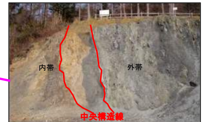
中央構造線の北川露頭
