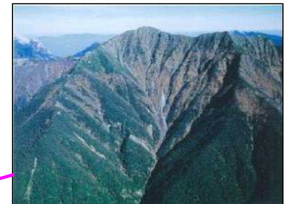
仙丈ヶ岳の崩壊状況
