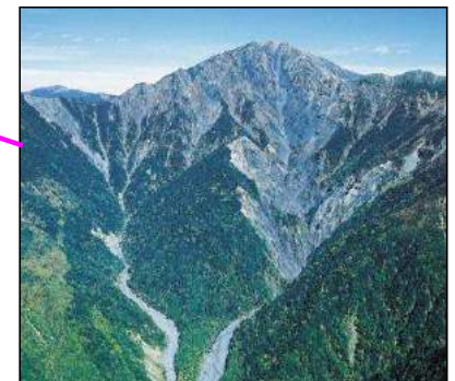
荒川大崩壊地
