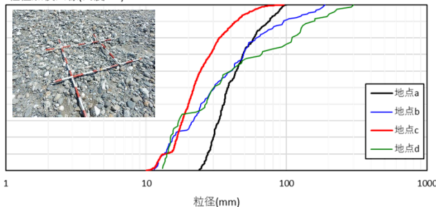
粒径加積曲線(高度5m)
